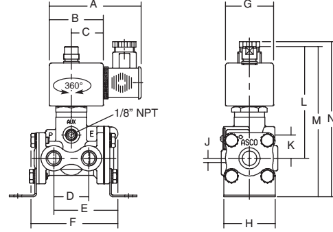
TYPE 04 Metal, epoxy coated / AISI 316 SS WP / WS: IEC 335 EM / WSEM: EN 60079-7/18 and EN 61241-1 WPIS / WSIS: EN/IEC 60079-11+26 / 61241-11
