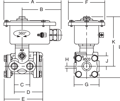
TYPE 06 Epoxy encapsulated PV: EN/IEC 60079-18 and EN/IEC 61241-18
