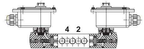
5/3 function
